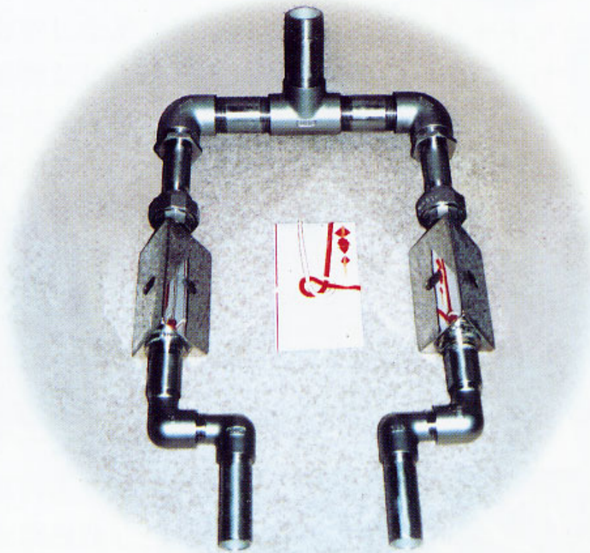
50m 3 受水槽用 エカロー・マシン装置/25A用2基
