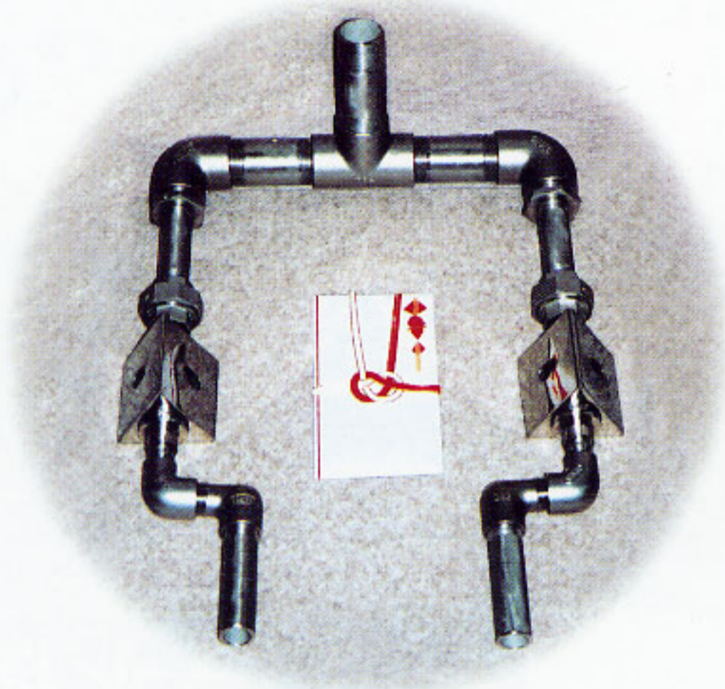
15m 3 受水槽用 エカロー・マシン装置/20A用2基
